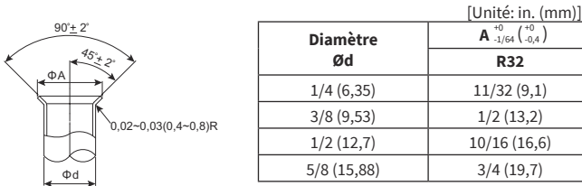
Figure 5.3 Traitement de l'évasement
